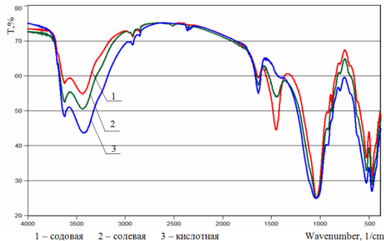
Рисунок 2 – ИК-спектры Милосского бентонита различных видов активации
