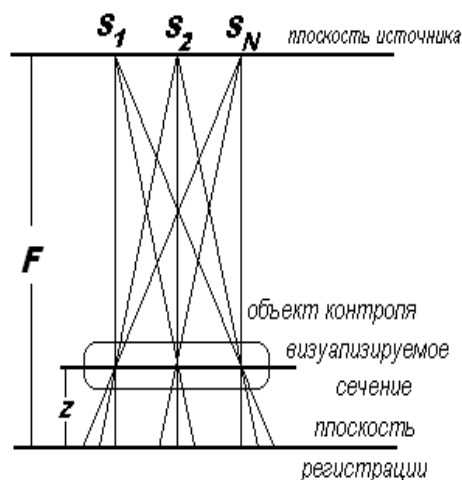
Рисунок 1- Регистрация проекций в классическом томосинтезе
