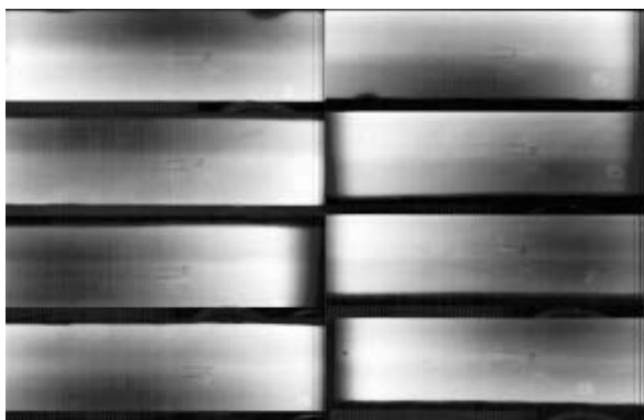
Рисунок 4- Радиографические проекции стального слитка
