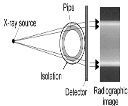
Рисунок 2 - Регистрация проекционных данных для томосинтеза (сканирование трубы)
