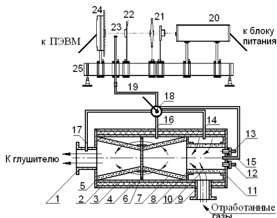
Рисунок 2 – Схема экспериментальной установки
