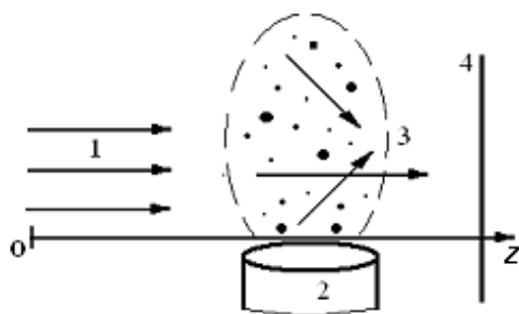
Рисунок 1 – Осевая схема записи голограммы микрочастиц
