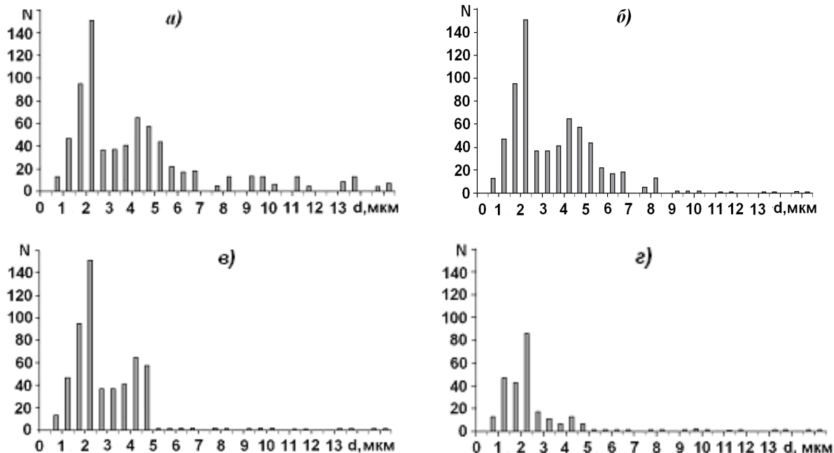
Рисунок 3 – Гистограмма распределения числа частиц по диаметрам: а) до каталитического нейтрализатора (КН); б) после прохождения первого элемента трехступенчатого КН; в) после прохождения второго элемента трехступенчатого КН; г) после прохождения трехступенчатого КН
