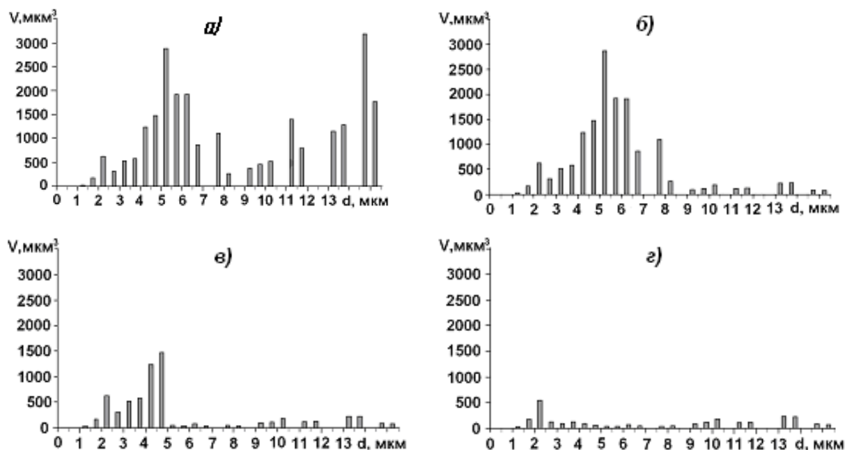
Рисунок 4 – Гистограмма распределения массы (объема) частиц по диаметрам: а) до КН; б) после прохождения первого элемента трехступенчатого КН; в) после прохождения второго элемента трехступенчатого КН; г) после прохождения трехступенчатого КН
