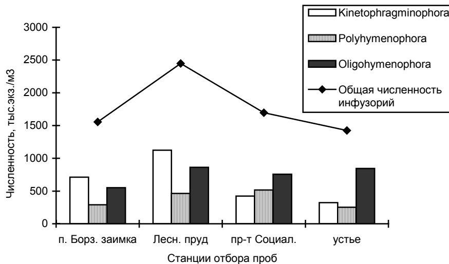
Рис. 1. Средняя численность различных групп инфузорий за период наблюдения май-октябрь 1997 г. на различных участках р. Барнаулки
