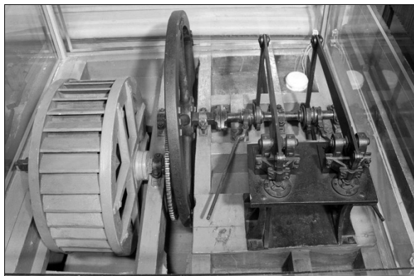
Рисунок 2 – Модель прорезного станка «Комар»
