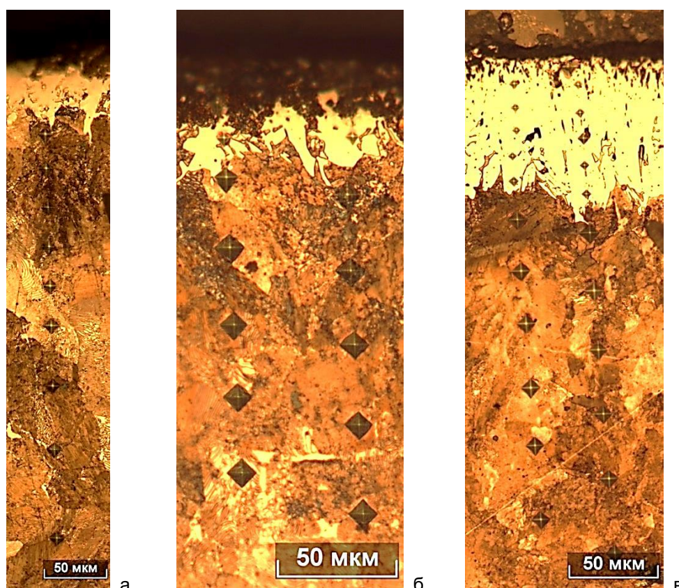
Рисунок 1 – Микроструктура диффузионных покрытий на стали У8А, полученных насыщением из различных смесей: а) № 1, б) № 2, в) № 3
