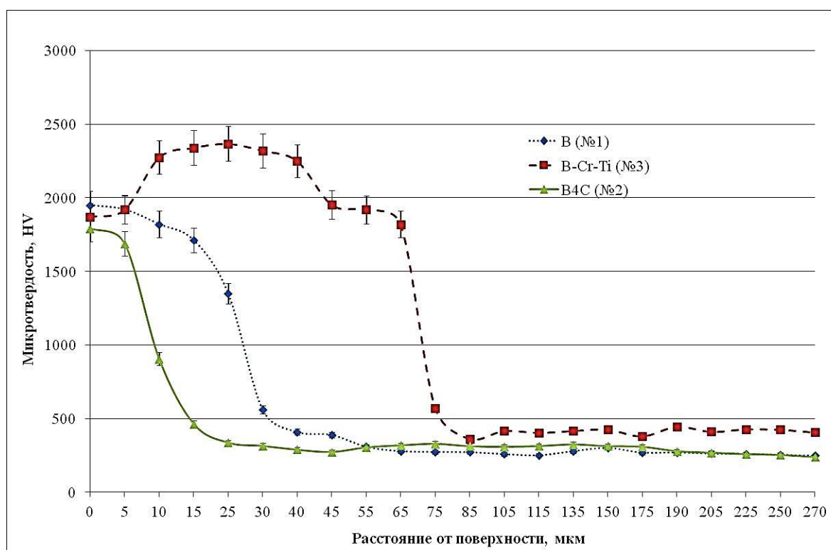
Рисунок 2 – Распределение микротвердости по сечению покрытий на стали У8, полученных диффузионным насыщением из различных насыщающих сред
