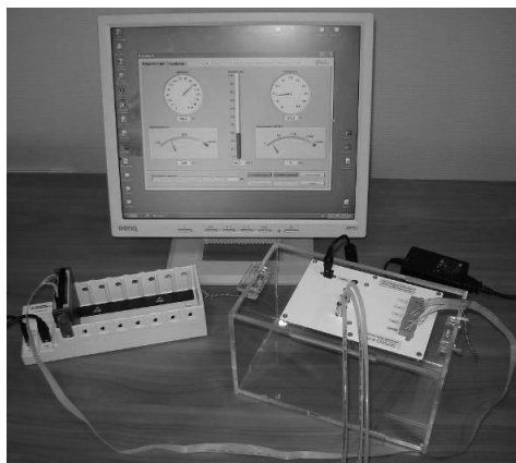
Рисунок 2 – Внешний вид лабораторного стенда
